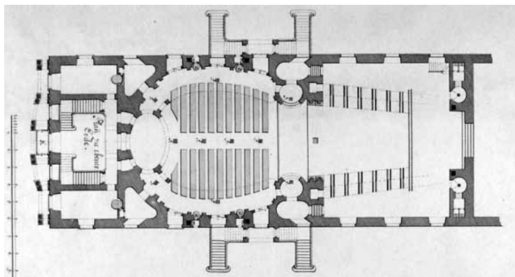
8. kép Az eszterházi operaház földszintű alaprajza. Joseph Ringer munkája 1789-ből. Országos Levéltár, T2 No. 1222-2.
